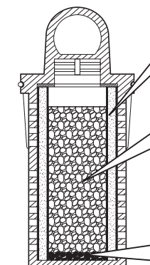
カートリッジ断面図
